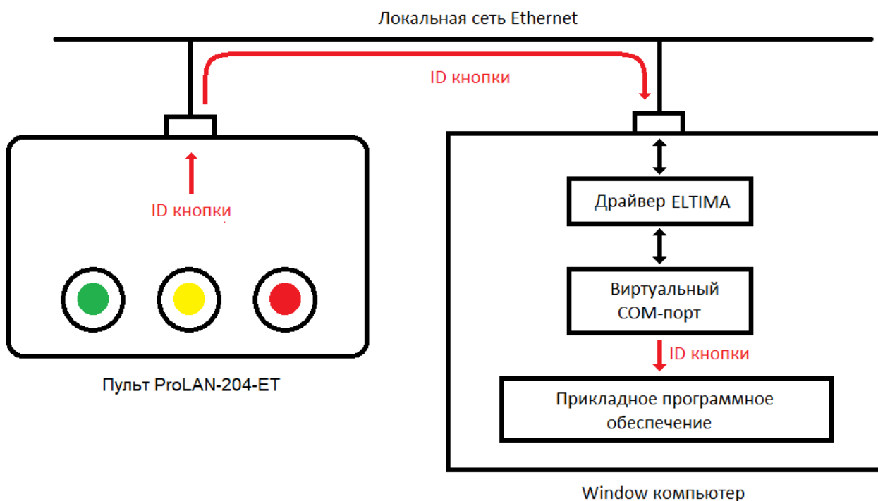
Рис. 9. Передача идентификатора нажатой кнопки пульта через виртуальный Com порт.
