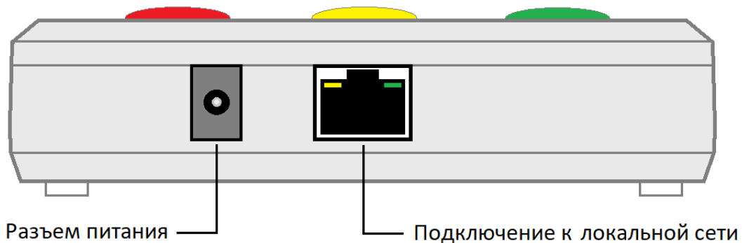
Рис. 1. Тыльная сторона пульта с разъемами подключения
